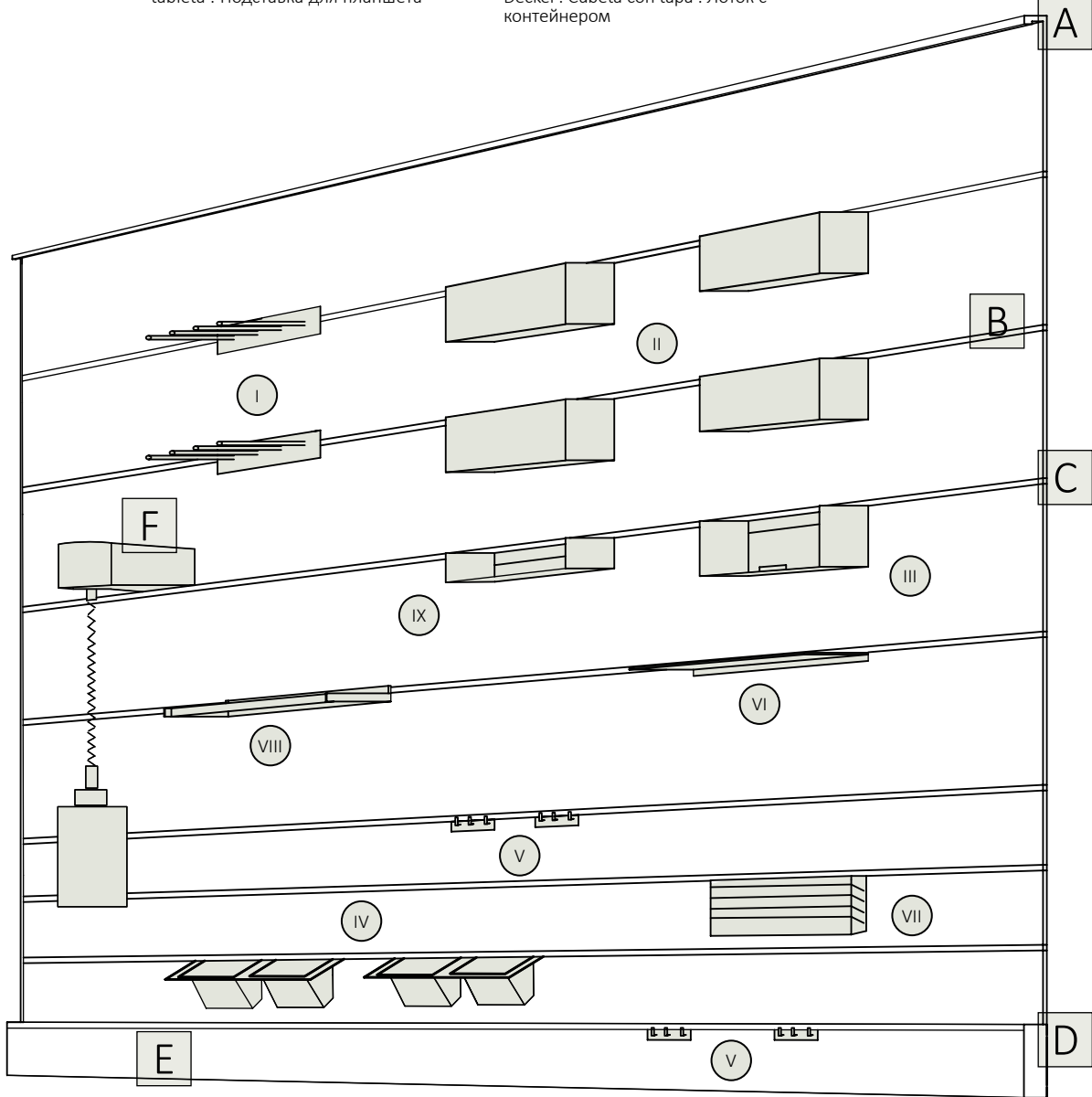
Porta tablet . Tablet shelf . Porte-tablette . Tablethalter . Soporte para tableta . Подставка для планшета
